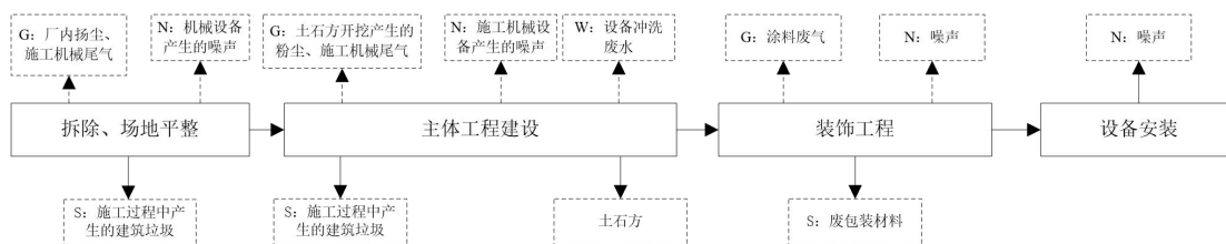
图 5-1 施工期工艺流程及产排污节点图
